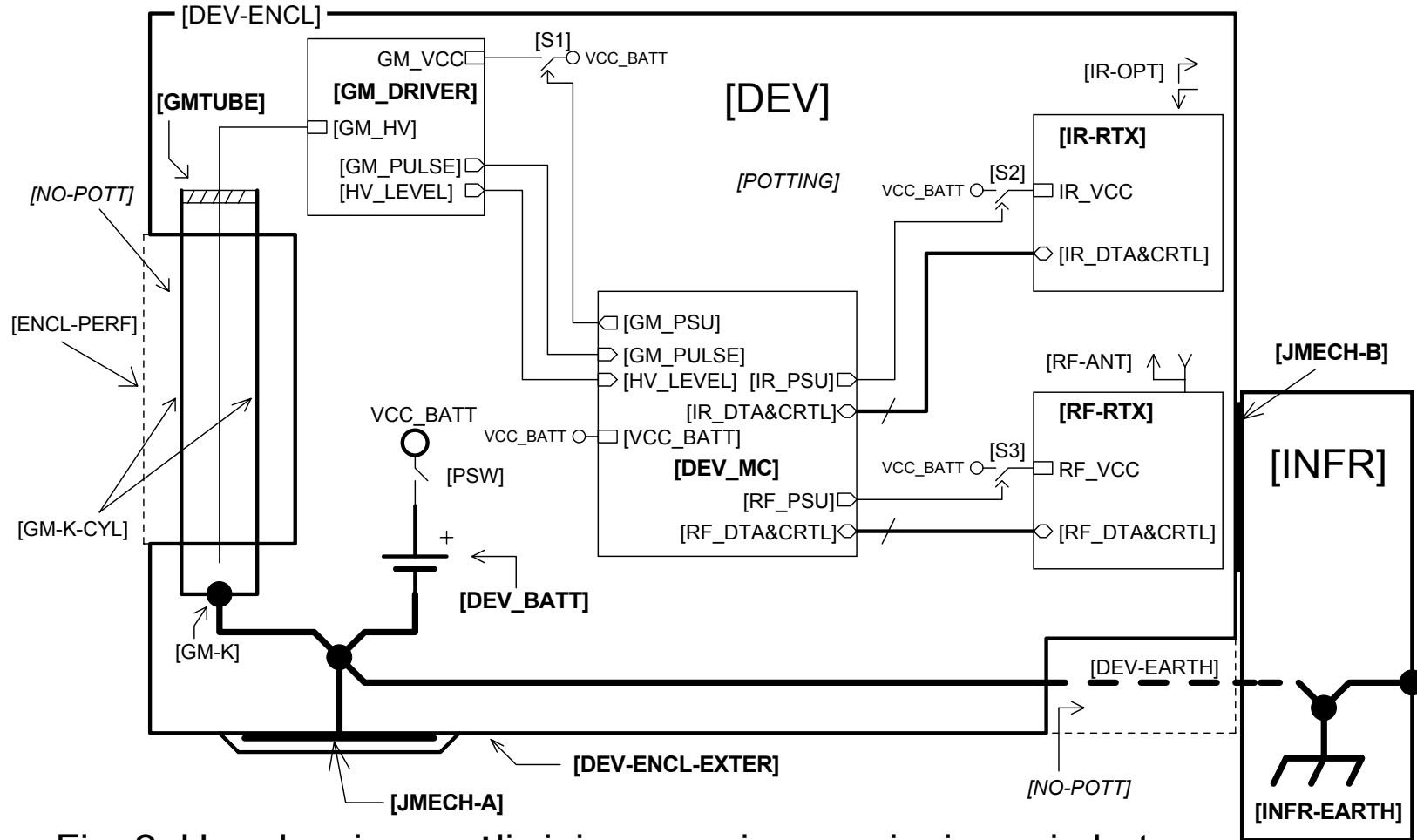
Fig. 2 Urządzenie umożliwiające pomiar promieniowania beta
